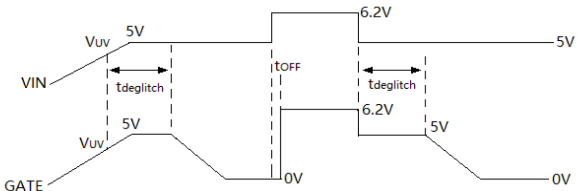
图 3 工作曲线
