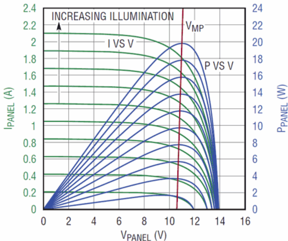
图2 CN3722实现光伏电池最大功率点跟踪
