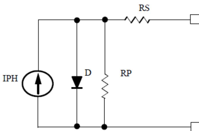
图 1 光伏电池简化电路模型
